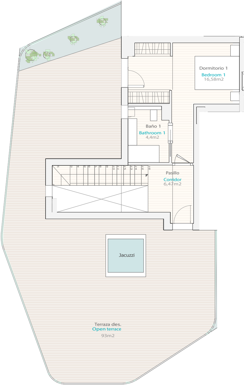
SOBREÁTICO | Penthouse
